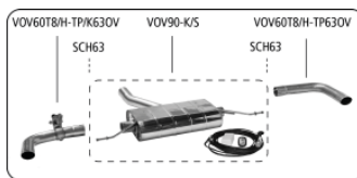
Twin Oval Ø 63 mm mit Abgasklappe / avec clapet d'échappement with exhaust flap / con válvula de escape
