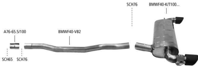
Twin RACE Ø 100 mm für Serienklappensteuerung avec clapet d'échappement with exhaust flap con válvula de escape
